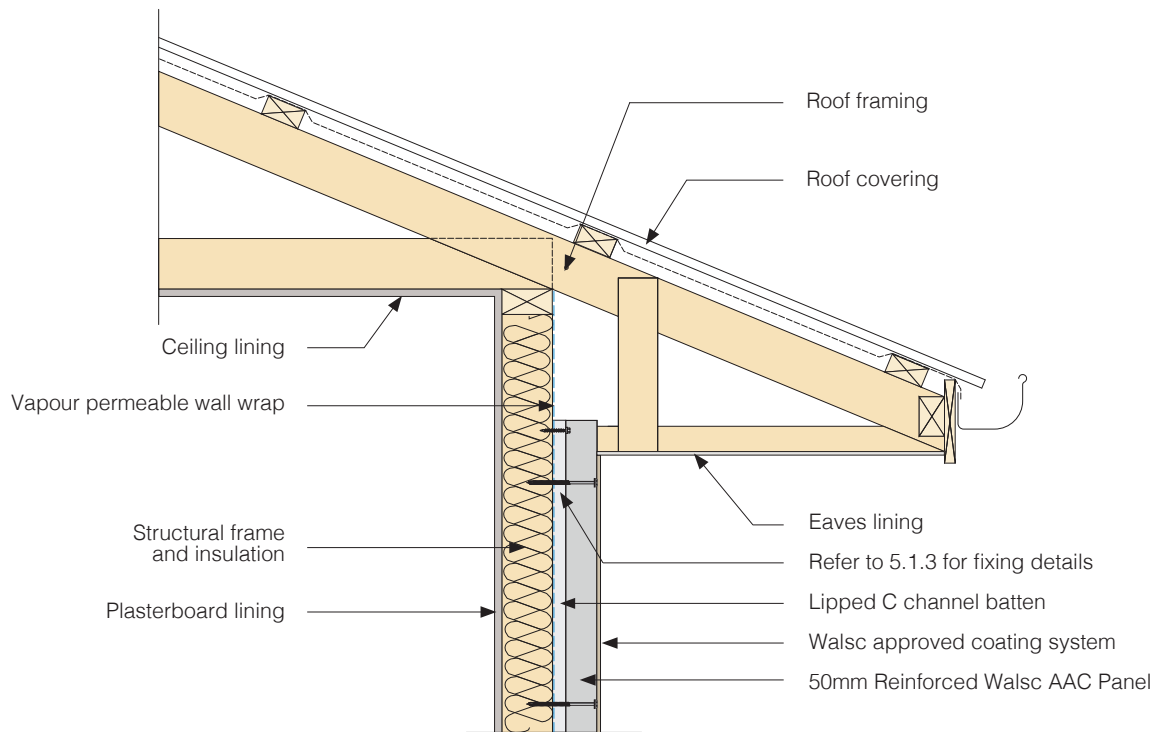
Fig 30. Eaves Detail 1
