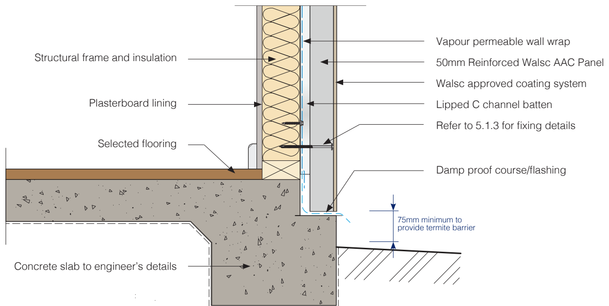
Fig 32. Slab Edge Detail
